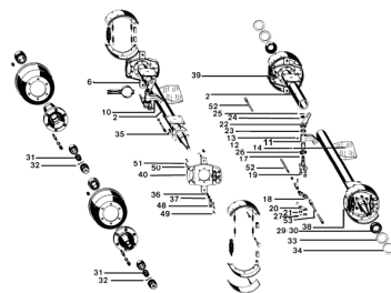
ETB-011565, Marka osi Berg. Oś ham. RS 5508 420x120, rozstaw kół 1800 mm, 8 otworów, 80 km/h (1/2)
