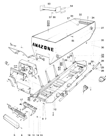
ETB-011544, Rama, szybkozłączce mechanizmu rozsiewającego, skrzynia
