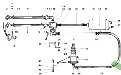
ETB-011572, Dwuobwodowy
