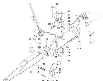
ETB-011548, Dyszel pociągowy z urządzeniem najazdowym AVE H 80 (1/2)
