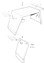
ETB-011600, Błotniki, osłony przeciwbłotne
