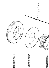
ETB-011571, Oś toczna skrętna GST-K 6006 w połączeniu z osią hamowaną ER 6506, ogumienie
