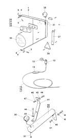
ETB-011554, Instalacja oświetleniowa
