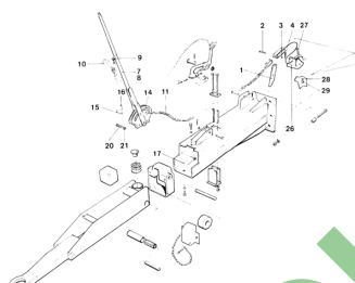
ETB-011549, Dyszel pociągowy z urządzeniem najazdowym AVE H 80 (2/2)
