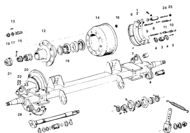
ETB-011564, Oś hamow. Peitz SSERD 8008, 420x180, rozstaw kół 1980 mm, 8 otworów, 80 km/h do ZG-B 8000 (2/2)
