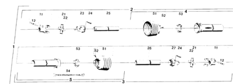
ETB-011575, Wałek przekładnikowy W 2300-SC15-1010
