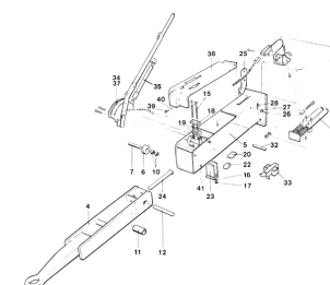
ETB-011551, Dyszel pociągowy z urządzeniem najazdowym AER H 80
