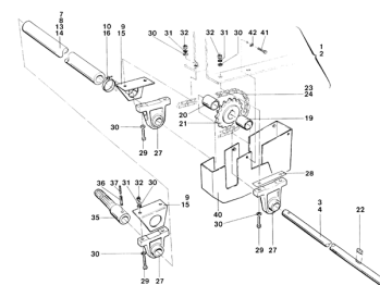
ETB-011574, Wałek napędu
