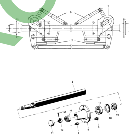
ETB-011570, Oś toczna skrętna GST-K 6006 w połączeniu z osią hamowaną ER 6506
