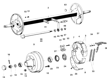
ETB-011568, Oś hamowana Peitz ER 8008, Brem. 310 x 80 do ZG-B z automatyką cofania, rozstaw kół 1970 mm
