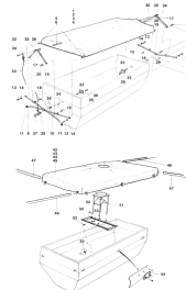
ETB-011602, Składana plandeka z ramą odchylaną, z króćcem zasypowym
