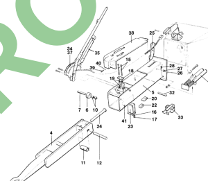
ETB-011550, Dyszel pociągowy z urządzeniem najazdowym AER 80
