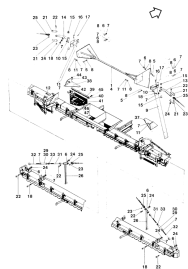
ETB-011588, Zawieszenie do ślimaka rozsiewającego ZG-B
