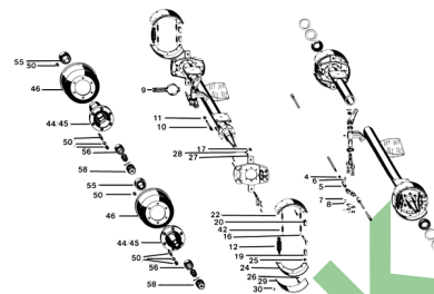
ETB-011566, Marka osi Berg. Oś ham. RS 5508 420x120, rozstaw kół 1800 mm, 8 otworów, 80 km/h (2/2)
