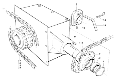
ETB-011596, Sprzęgło do napędu od koła jezdnego
