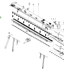
ETB-011591, Wysięgnik do ślimaka rozsiewającego (1/2)
