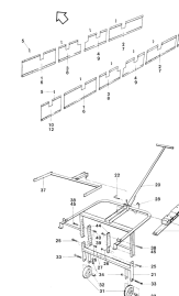
ETB-011595, Zaslona przeciwpylowa
