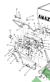
ETB-011546, Zasuwa
