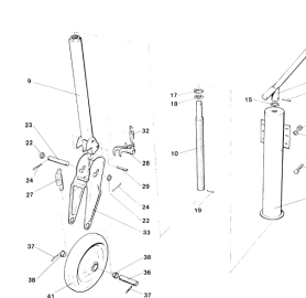
ETB-011555, Koło podporowe
