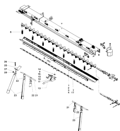
ETB-011592, Wysięgnik do ślimaka rozsiewającego (2/2)
