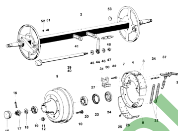
ETB-011569, Oś hamowana Peitz ER 6506, Brem. 310 x 80 do ZG-B z automatyką cofania, rozstaw kół 1900 mm
