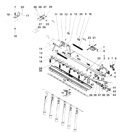
ETB-011593, Wysięgnik końcowy do ślimaka rozsiewającego (1/2)
