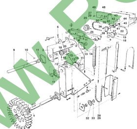
ETB-011597, Napęd od koła jezdnego
