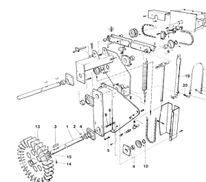
ETB-011599, Napęd od koła jezdnego (wałek koła jezdnego)
