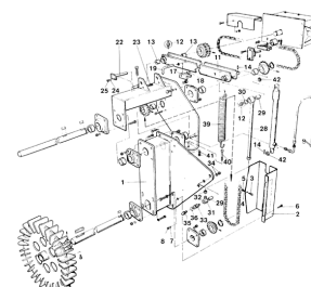
ETB-011598, Napęd od koła jezdnego (rama odchylana)
